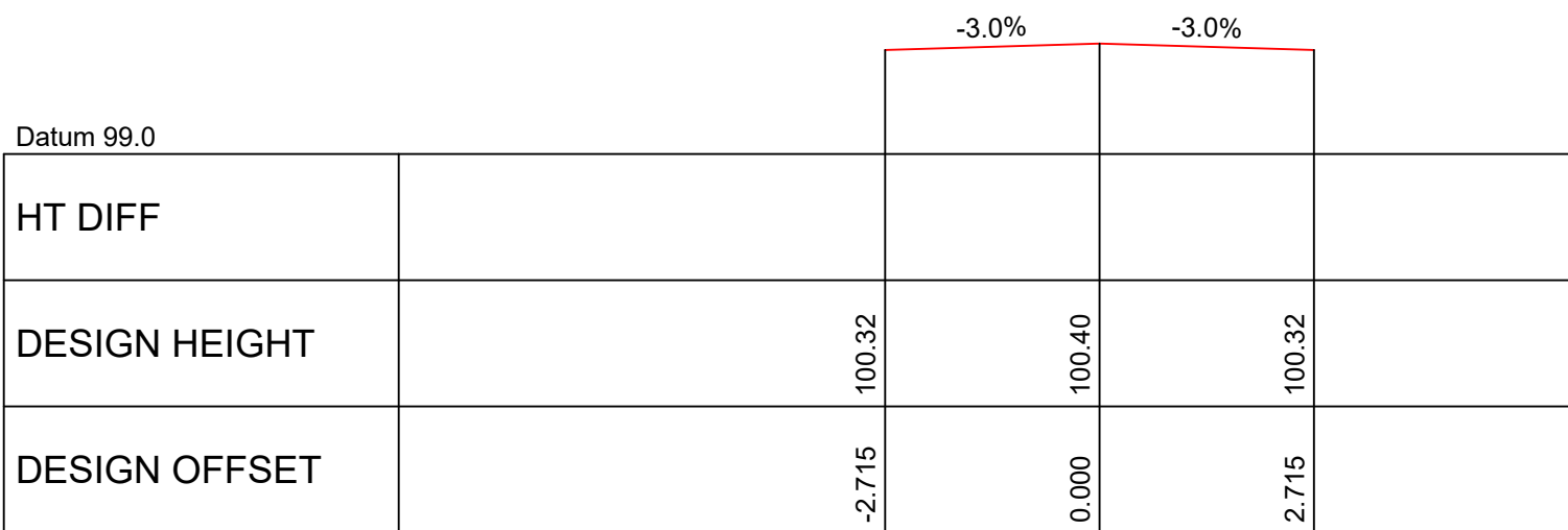
CHAINAGE 20.000
