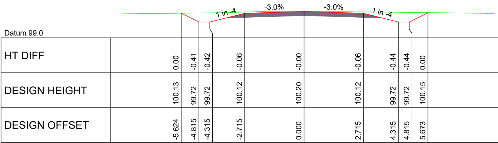
CHAINAGE 40.000
