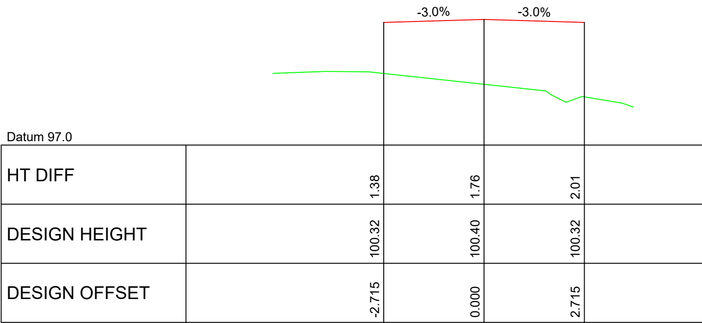
CHAINAGE 15.000
