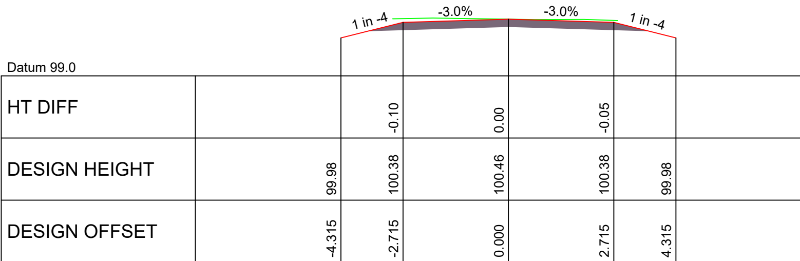
CHAINAGE 0.000
