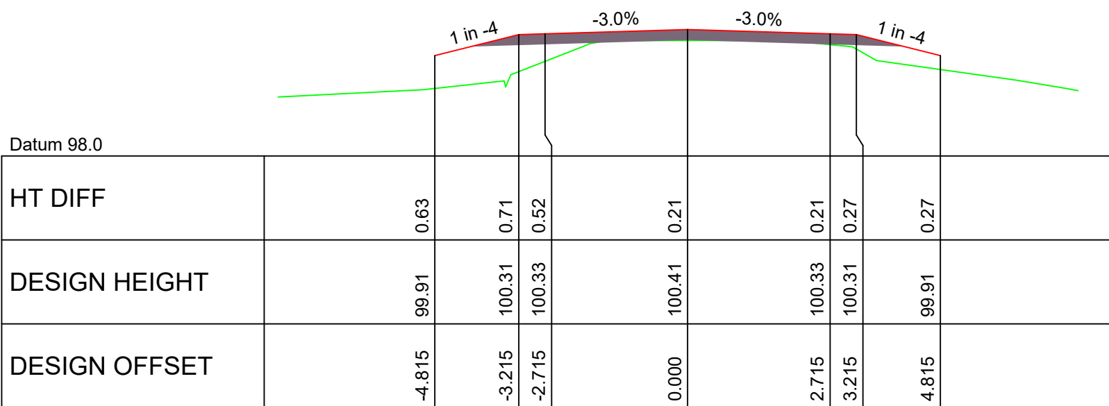
CHAINAGE 10.000
